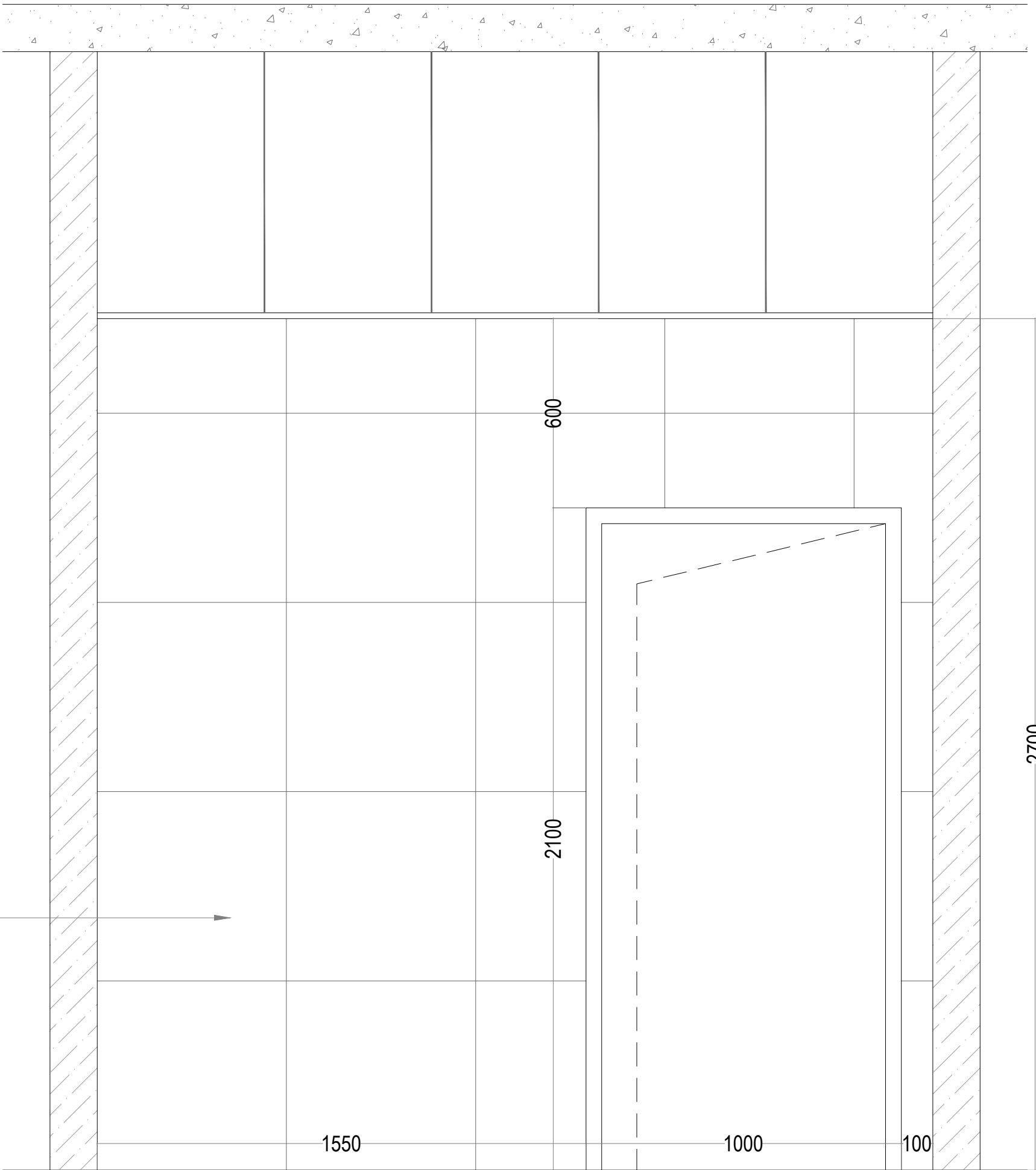
ELEVATION -03
