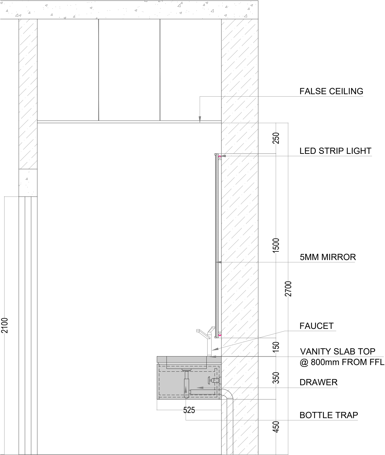
ELEVATION -04
